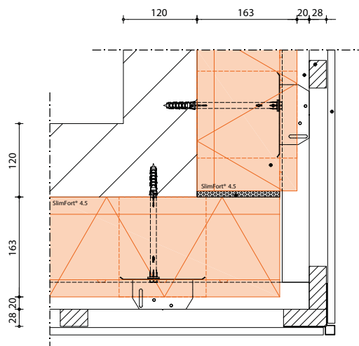
Voorbeeld detaillering horizontale aansluiting bij een buitenhoek
