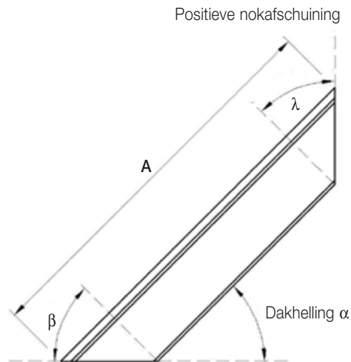
Positieve gootafschuining
