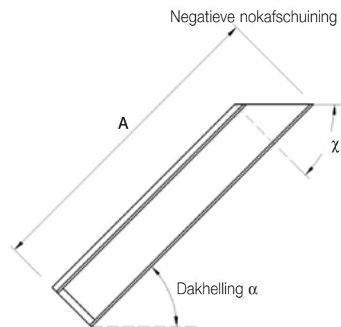
Standaard: recht, met houten gootregel
