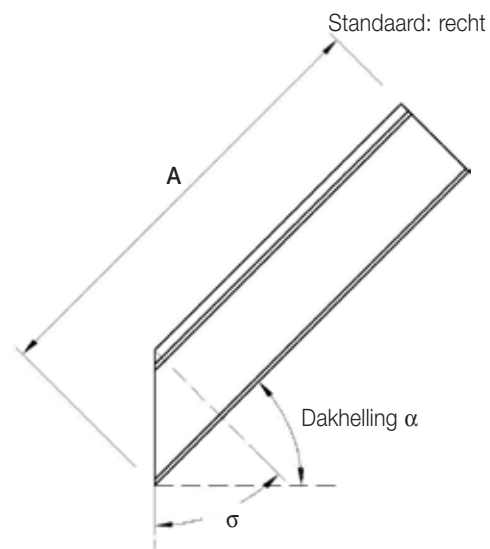
Negatieve gootafschuining
