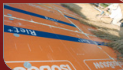
↑ IsoBouw Riet* - Schroefdakelement voor rietbedekking - Élément de toit à visser pour une couverture en chaume
